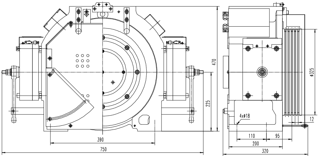
附 1：Mini.6 系列无齿曳引机的外形安装尺寸
