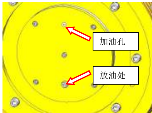
图 7 轴承注脂孔位置
