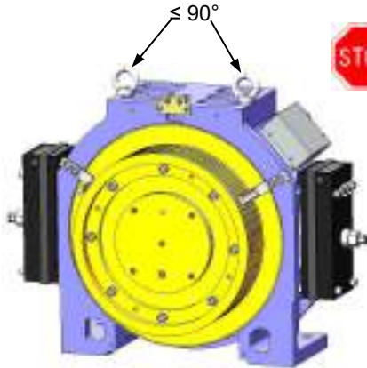
图 2 产品吊装示意图
