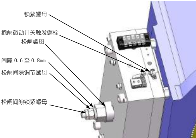
图 6 松闸螺母及抱闸微动开关结构示意图
