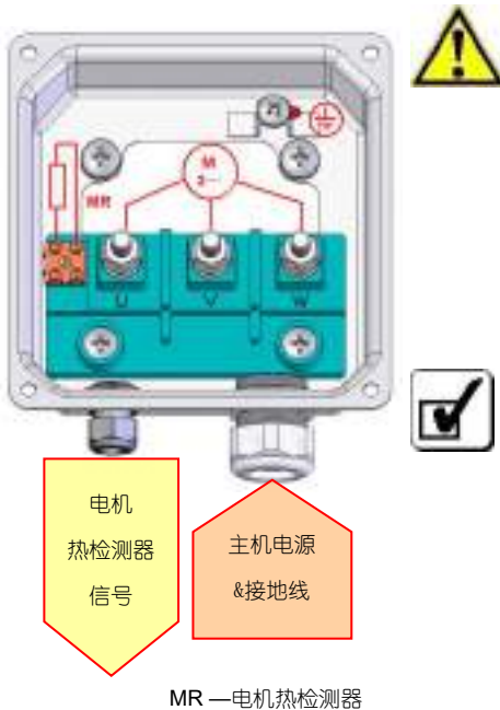
图 3 主机接线盒的接线示意图
