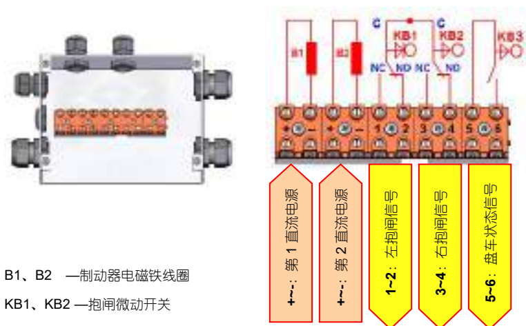
b. 用户电源为直流双电压的接线示意图
