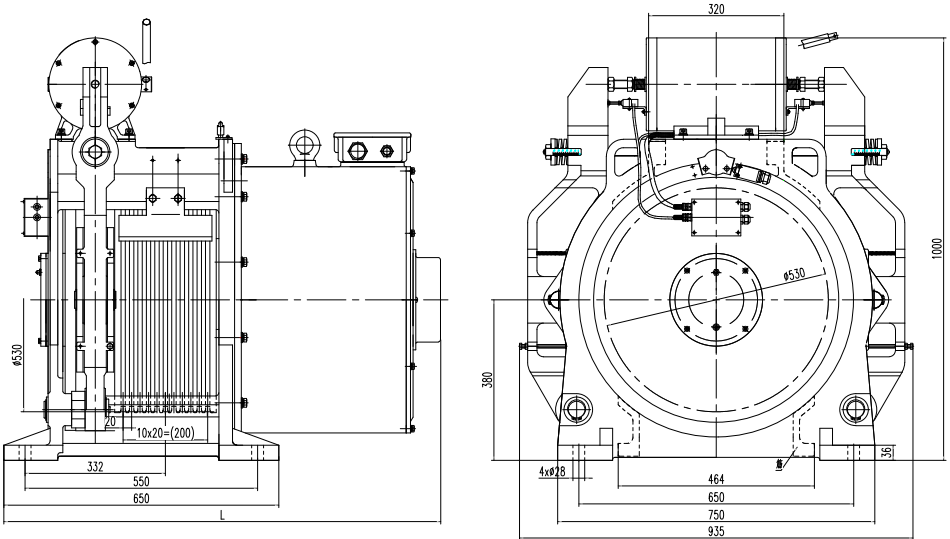
附 1：WTYF380 系列无齿曳引机的外形安装尺寸和机电参数
