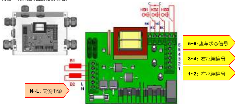
a. 用户电源为交流单电压的接线示意图
