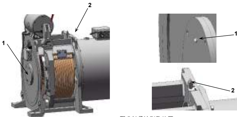
图 5 轴承注脂孔位置
