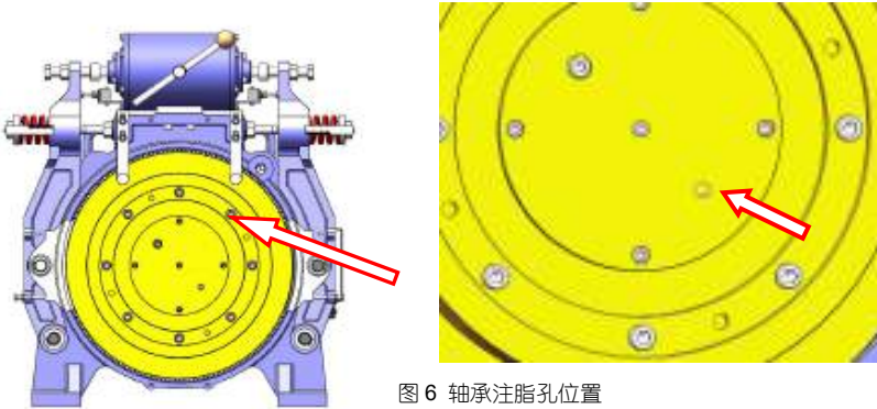
图6 轴承注脂孔位置
