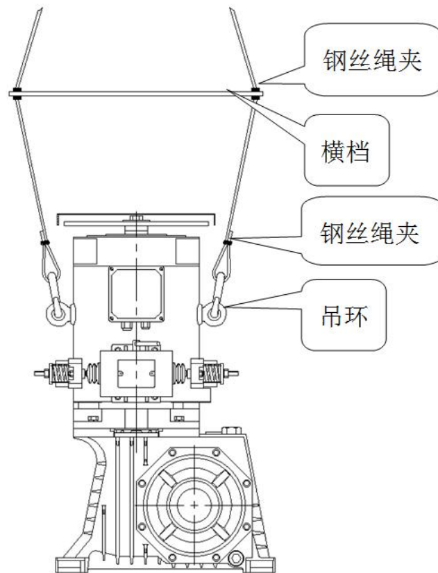
图 2 吊装示意图
