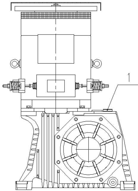
图 4 主机的润滑示意图
