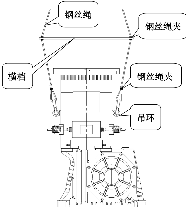
图 2 吊装示意图
