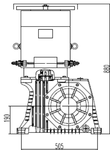
扶梯主机外形安装尺寸图
