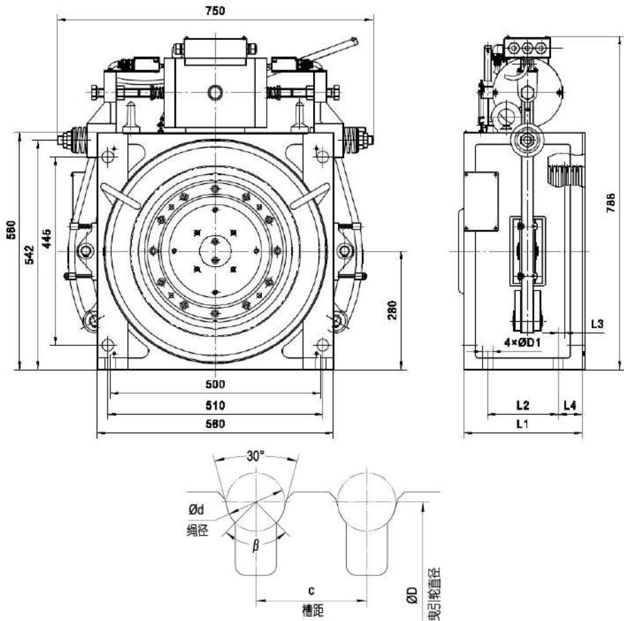
附 1：WWTY 系列无齿曳引机的外形安装尺寸
