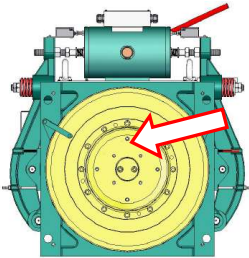
当注油孔在前端时，取掉其上的闷盖，将孔转至图示竖直位置，油枪插入油杯中注油
