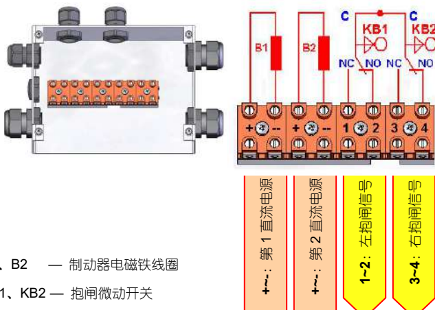
b. 用户电源为直流双电压的接线示意图
