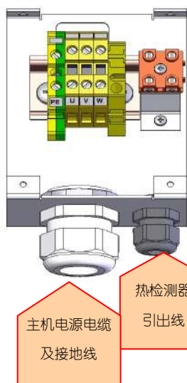
图 3 主机接线盒的接线示意图
