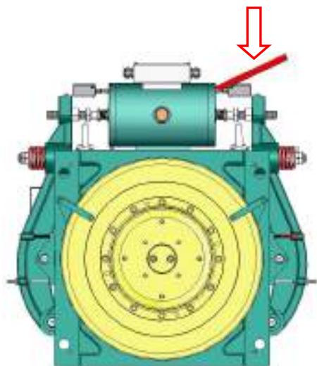
手动松闸
