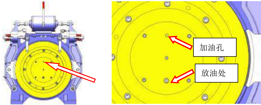
图6 轴承注脂孔位置
