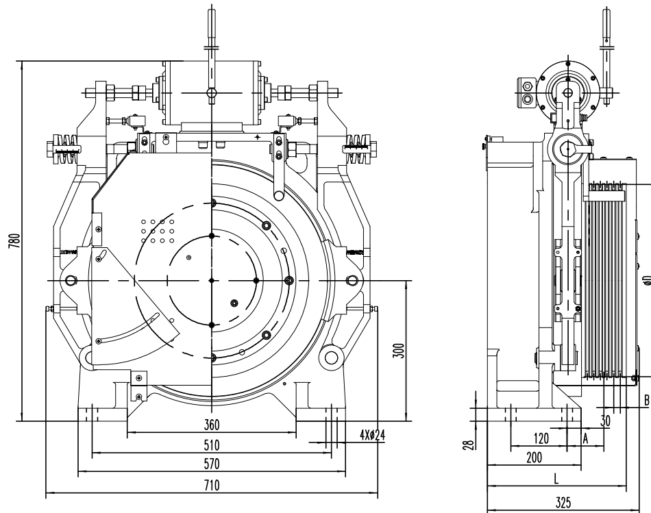
附 1：WWTY.5A/C 系列无齿曳引机的外形安装尺寸
