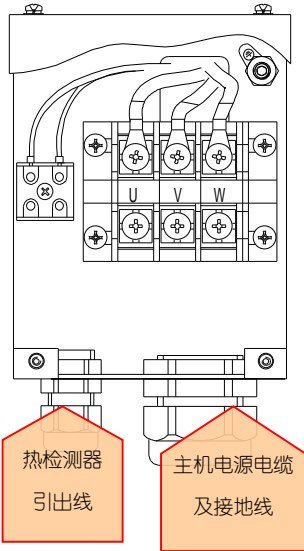
图 3 主机接线盒的接线示意图
