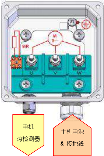
图 3 主机接线盒的接线示意图 MR —电机热检测器
