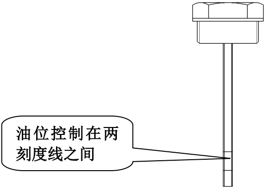
图 4 油标示意图
